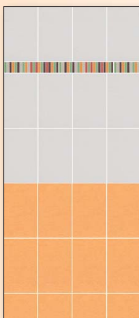
panel č. 28 Behappy White/Orange výška panelu 2301 mm koupelna doplatek: 1720 Kč/bm WC doplatek: 2150 Kč/bm
