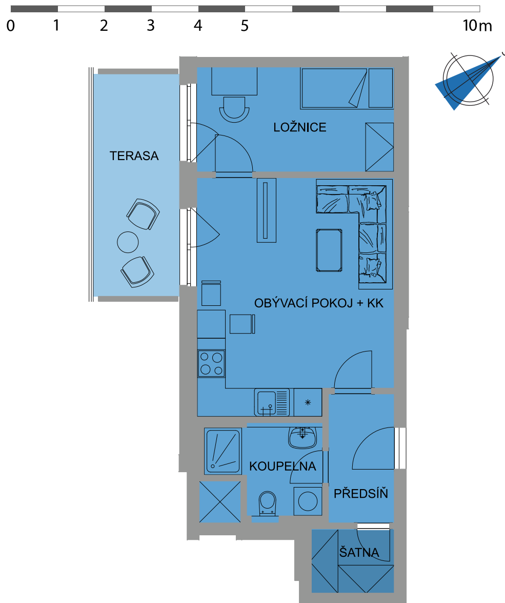
Půdorys podlaží
