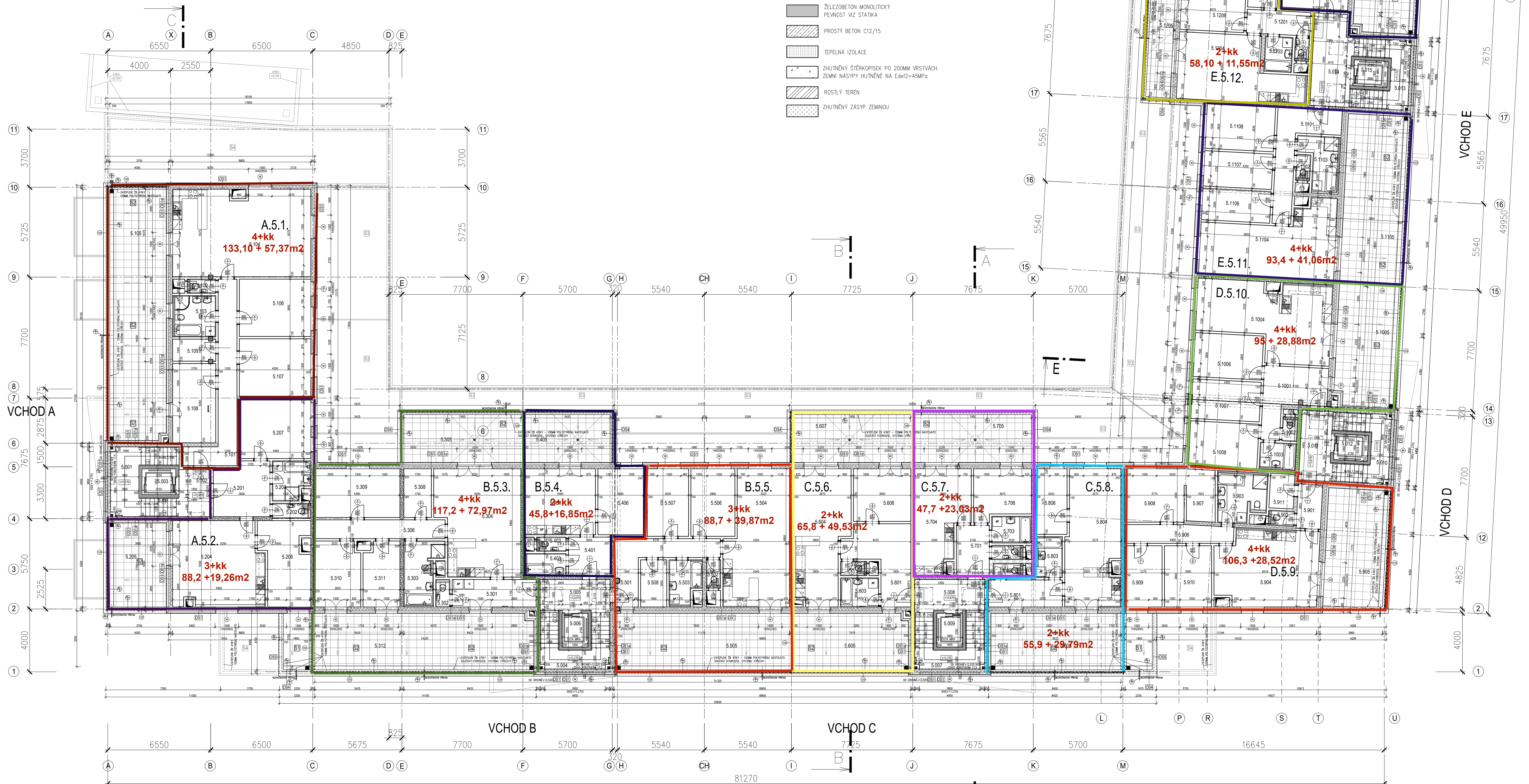
PŮDORYS 5.NP 1:100
