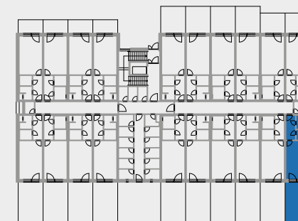
Půdorys podlaží/Floor Plan
