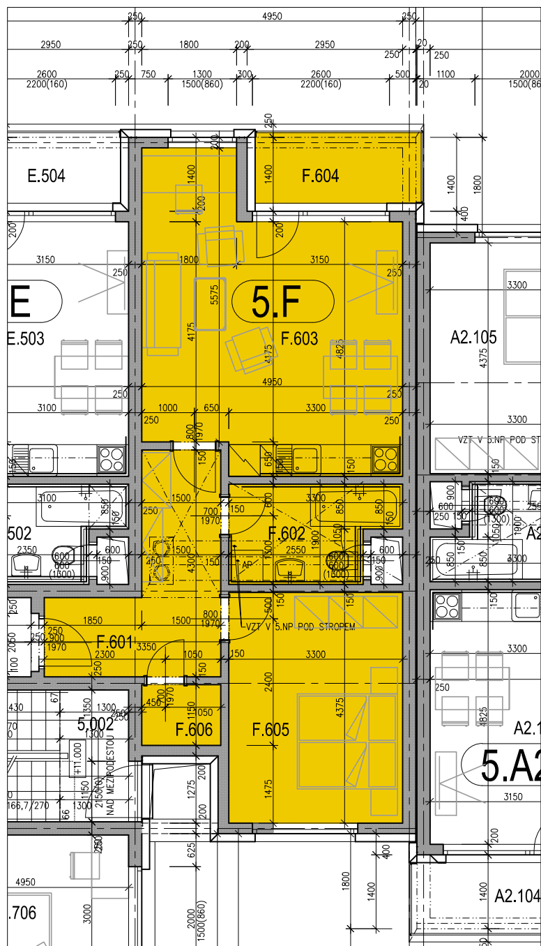
SCHEMA DOMU A1 - PŮDORYS 5.NP
