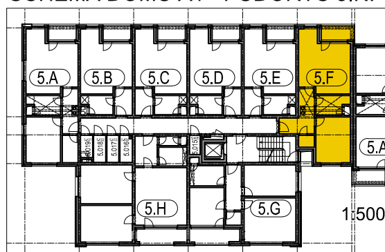
SCHEMA DOMU A1 - PŮDORYS 5.NP
