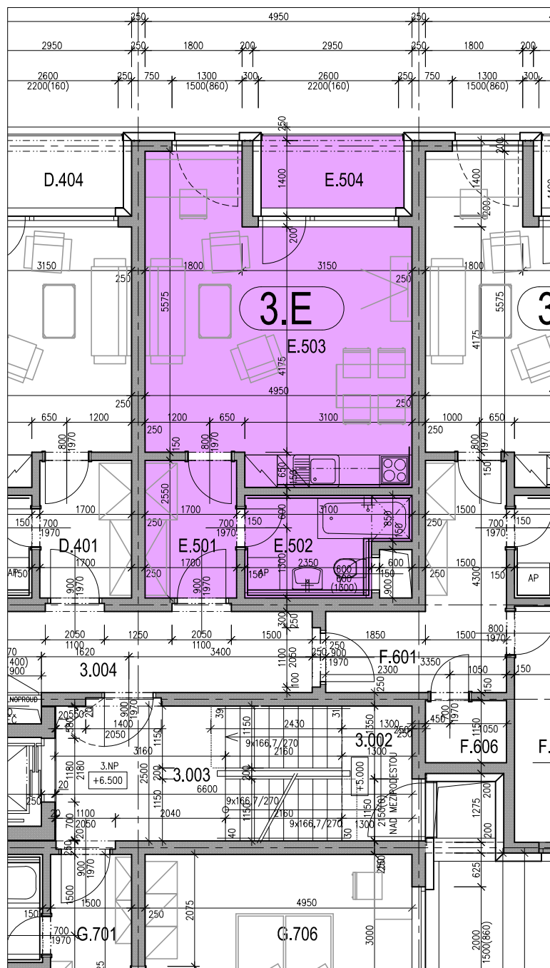
SCHEMA DOMU A1 - PŮDORYS 3.NP
