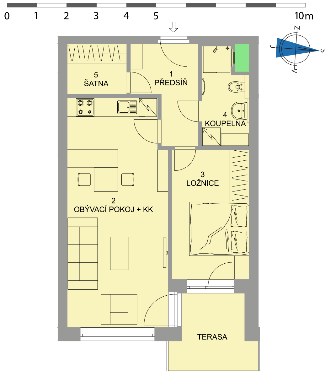
Půdorys podlaží/Floor Plan
