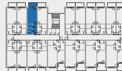
Půdorys podlaží/Floor Plan
