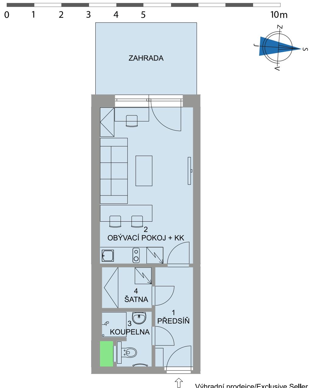
Půdorys podlaží/Floor Plan
