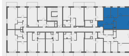
Půdorys podlaží/Floor plan
